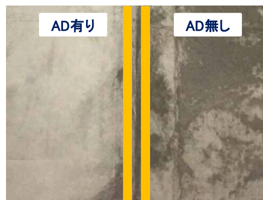
経年後のコンクリートの表面状況
